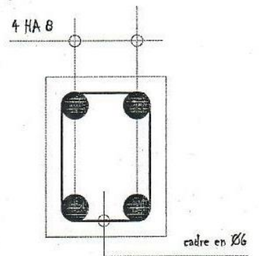
detail linteau de 15 x 20
