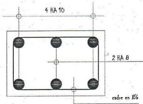
detail amorces de 20 x 30
