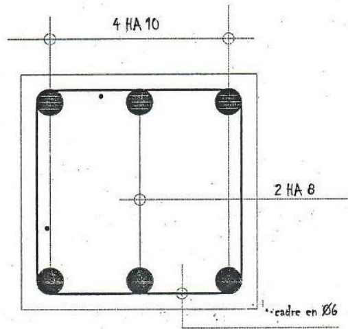
detail poutres de 30 x 30
