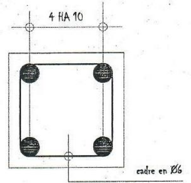
detail longrine de 20 x 20
