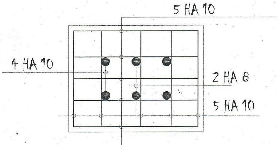
detail semelles de 40 x 50
